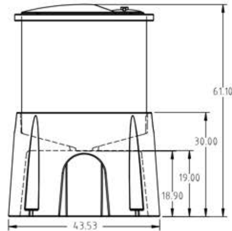
DC036-STP POLY STAND
