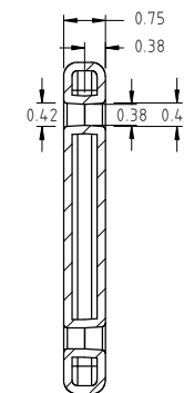
SECTION A-A SCALE 1:3
