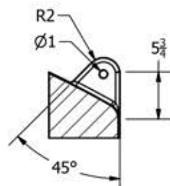
SECTION A-A SCALE 1:12
