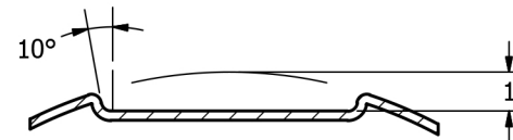
SECTION A-A SCALE 1:4
